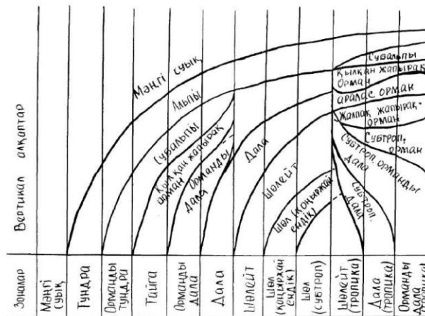
Сурет 24. Континенттегі табиғи зоналардың үстіндегі вертикал алқаптардың үлгісі (Макаев, 1954)
