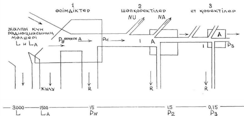
Сурет 18. Қауымдағы энергия тасымалдануының қарапайым диаграммасы. 1-продуценттер-автотрофтар; 2-бірінші консументтер-фитотрофтар; 3-екінші консументтер-саркотрофтар. L және L_A жалпы және сіңірілген күн радиациясы; P_g және P_n - жалпы және таза өнім, A - Ассимиляцияланған энергия; N_A және N_U ассимиляцияланбаған және пайдаланбаған энергия; R - тыныс алу кезінде жоғалған энергия; төмен жағындағы - 1 \text{ м}^2 жерге түскен 3000 ккал энергияның тасымалдануындағы өзгеруі көрсетілген (Одум, 1968).
